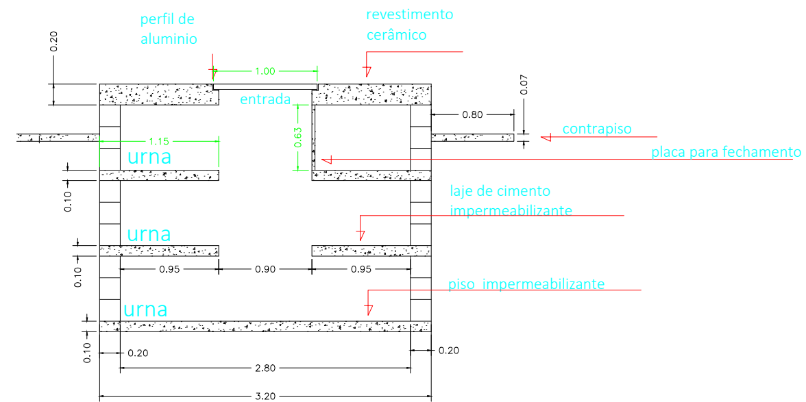
CORTE BB (elevação frontal) ESC 1:50
