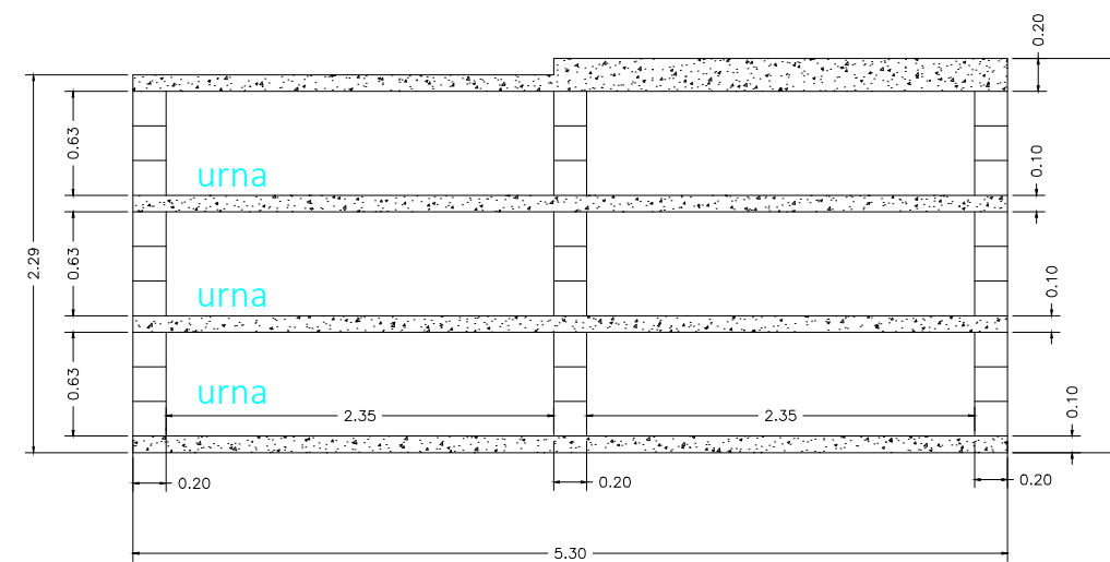
CORTE AA (elevação lateral) ESC 1:50
